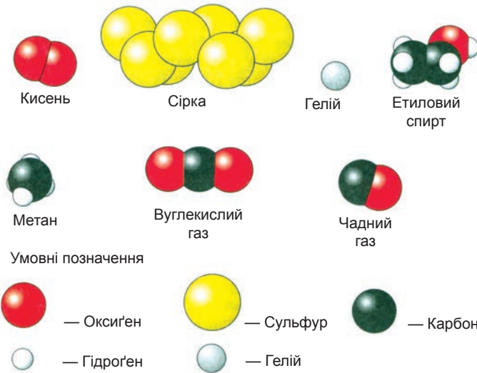
Мал. 44. Моделі молекул деяких речовин
