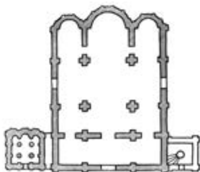
Успенский собор Киево-печерской лавры (реконструкция и план)
