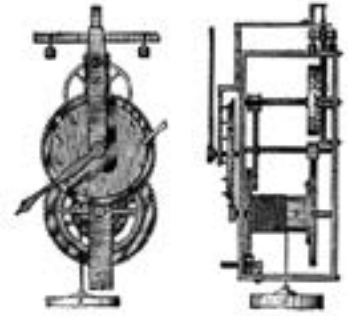
Часовой механизм
