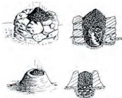
Реконструкція горнів для плавлення мідної руди у носіїв зрубної культури. Автори А. Копил, С. Татарінов
