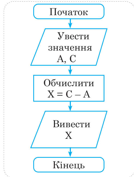
Рис. 21. Способи опису алгоритмів
