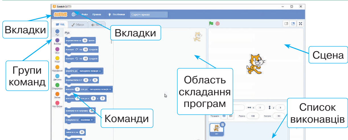
Рис. 19. Будова вікна програми Scratch
