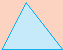
Гострокутний трикутник
