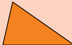
Різносторонній трикутник (усі сторони різні)
