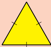
Рівносторонній трикутник (усі сторони рівні)
