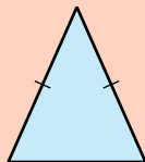
Рівнобедрений трикутник (дві сторони рівні)
