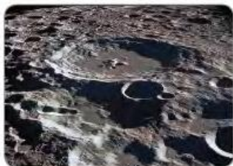
Кратери Місяця
