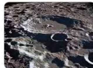
Кратери Місяця
