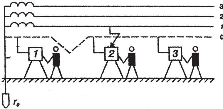
Рис. 13. Трифазова електрична мережа з глухозаземленою нейтраллю та пошкодженим нульовим проводом
