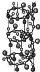
вторинна структура
