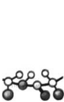
первинна структура
