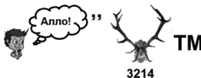
(Алгоритм)
