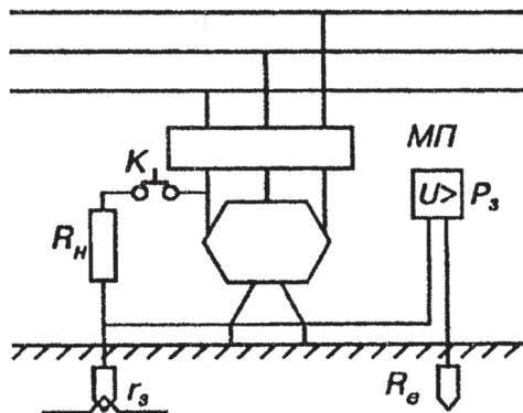
Рис. 10. Схема захисного вимкнення, що реагує на величину напруги корпусу електрообладнання стосовно землі
